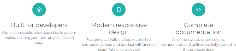
Figura 7 – Secção Icons
