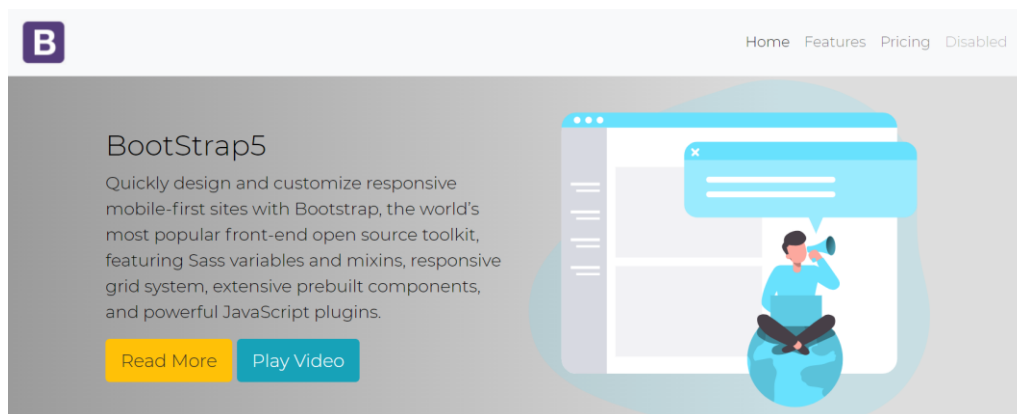
Figura 4 – Secção Header
